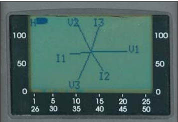
Three-phase diagram V1 V2 V3 I1 I2 I3 \varphi
